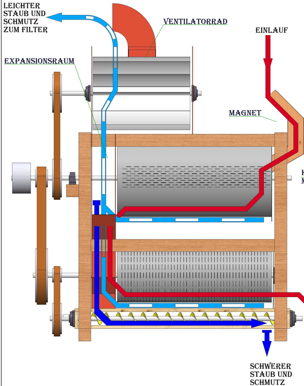
SCHEUERMASCHINE
